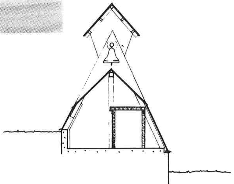
Foto: Klockstapeln sedd från öster 1997. (GSM 15-97,10) Sektion: Klockstapeln sedd från norr i samband med reparation 1990. Arbetsritning upprättad av DEFYRA Arkitekter AB. (Kyrkonämndens centralarkiv)
