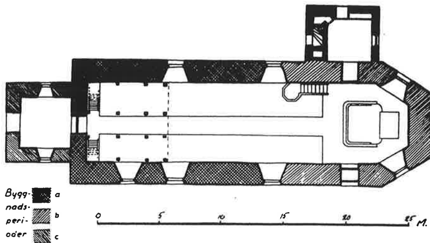
Fig. 21. Plan. Efter äldre original i A. T. A., kompletterat av S. Boëthius 1941. Skala 1:300. Grundriss. Plan.
