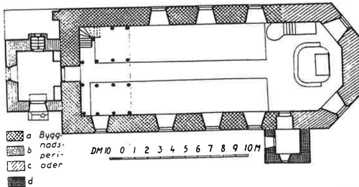
Plan. Uppmätt av W. Karlberg och I. Cruickshank 1931.
