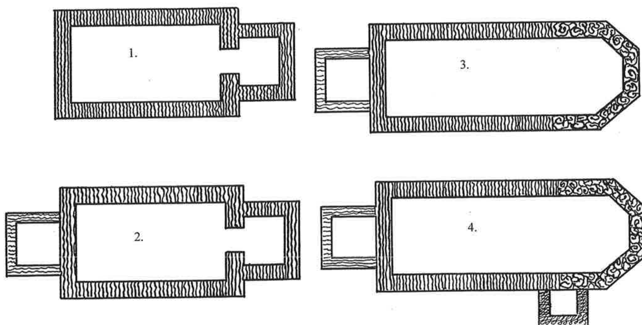
Plan över Torslanda kyrka och dess tillbyggnadsfaser. 1) ca 1200 2) 1766 3) 1780 4) 1806 (Hellström m fl.)
