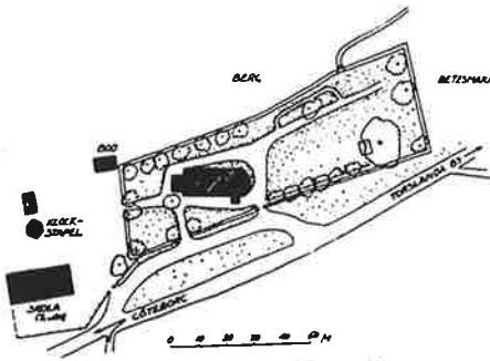
Situationsplan. Uppmätt av W. Karlberg och I. Cruickshank 1931, kompl. 1941 av S. Boëthius. Skala 1: 3 000. Lageplan. Plan of situation.
