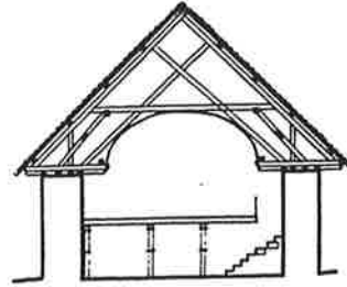
Tvärsnitt mot v. Uppmätt av W. Karlberg och I. Cruickshank 1931. Skala 1: 300.
