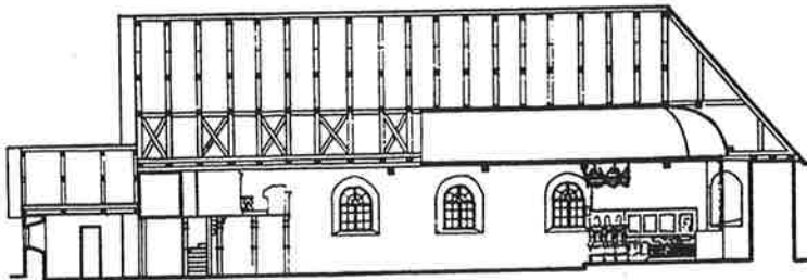
Längdsnitt mot n. Uppmätt av Wivi Karlberg och Ingeborg Cruickshank 1931. Skala 1: 300.
