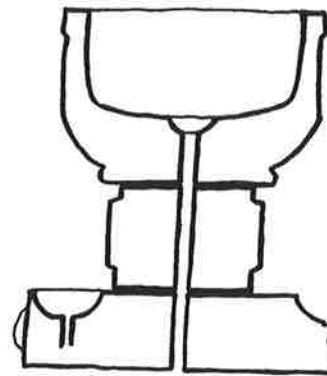
Fig. 19. Dopfunt i genomsnitt. Uppmätt av I. Cruickshank och W. Karlberg 1931. Skala 1:20.
