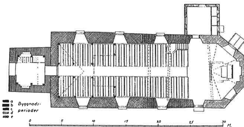
Fig. 5. Plan. Uppmätt av A. Funkquist 1928, kompletterad av S. Boethius 1941. Skala 1:300. Grundriss. Plan.
