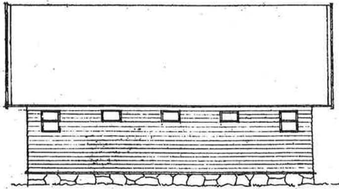
Fasad åt norr och söder
