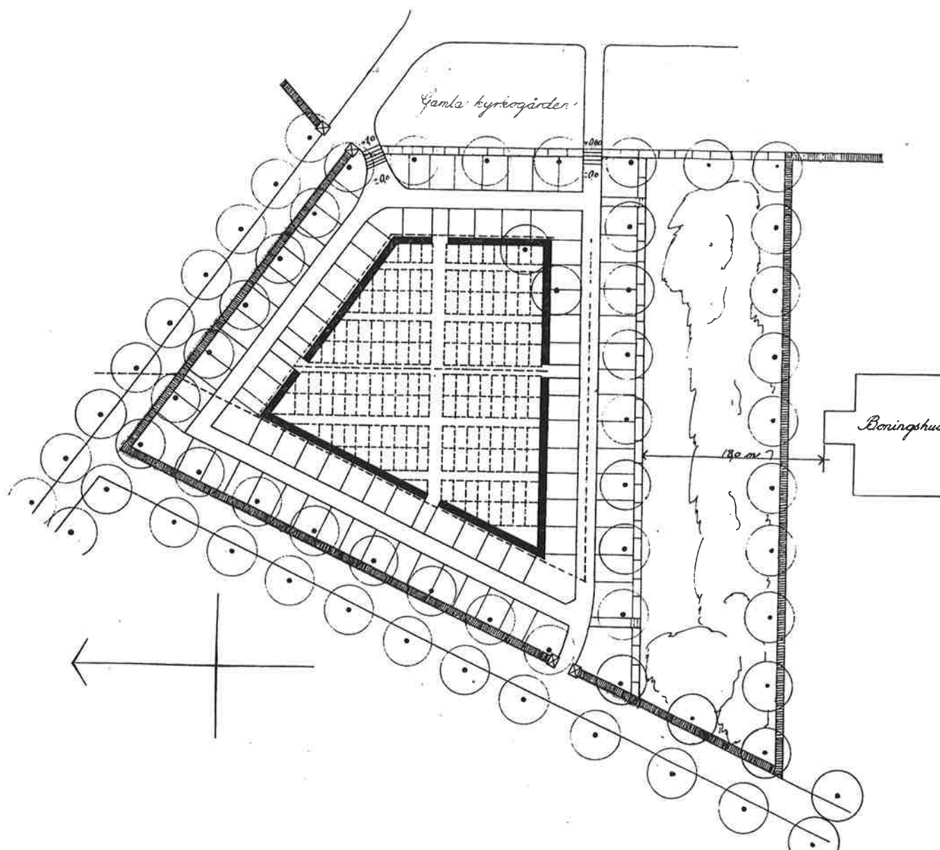
Förslag till utvidgning av Styrso kyrkogård upprättat 1929 av arkitekt Erik Friberger. (Styrso församlings arkiv)
