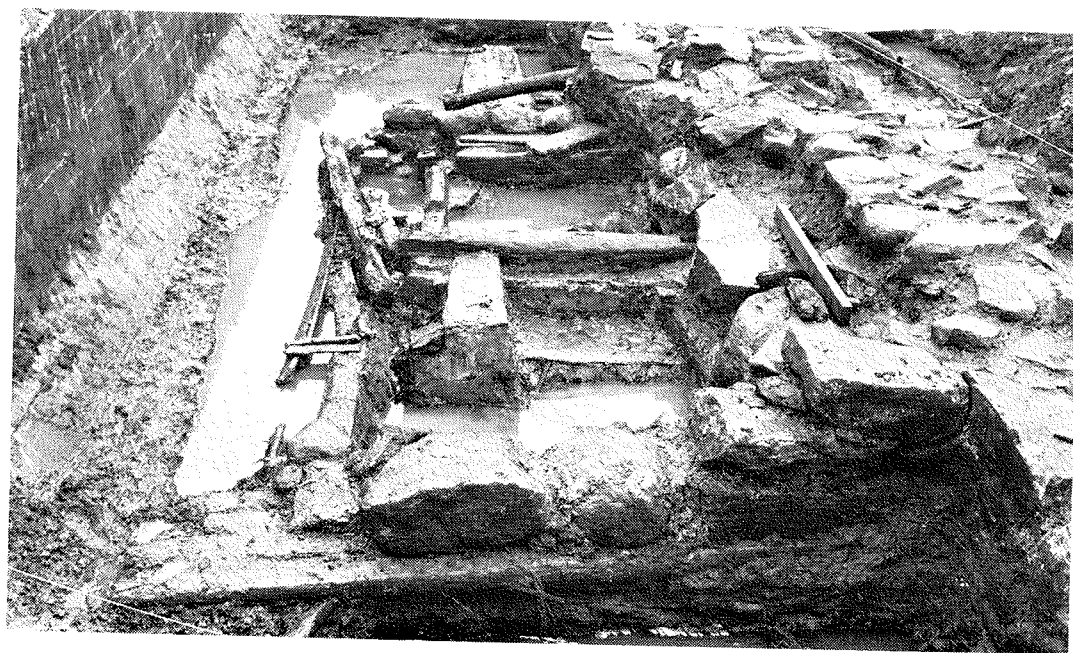
Fig.20, Kvarteret Enigheten, anl 3F. Foto mot norr. Foto EJ -79
