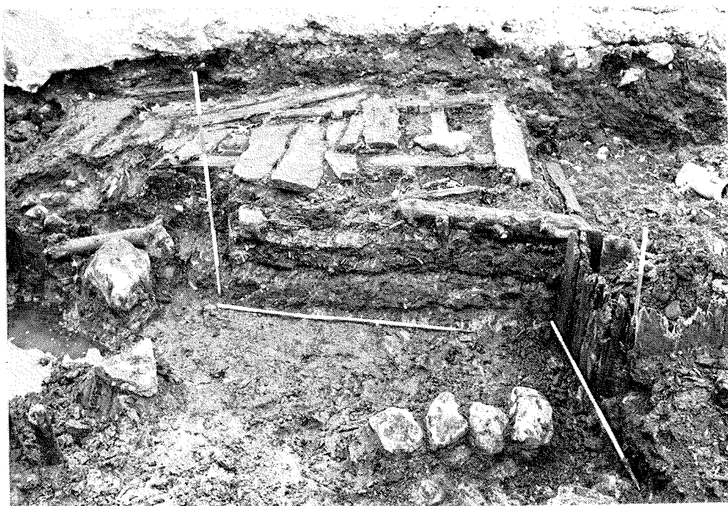
Fig. 32, Kvarteret Enigheten, anl 11. Golv och avfallsbinge. Foto mot väster. Foto: EJ -79
