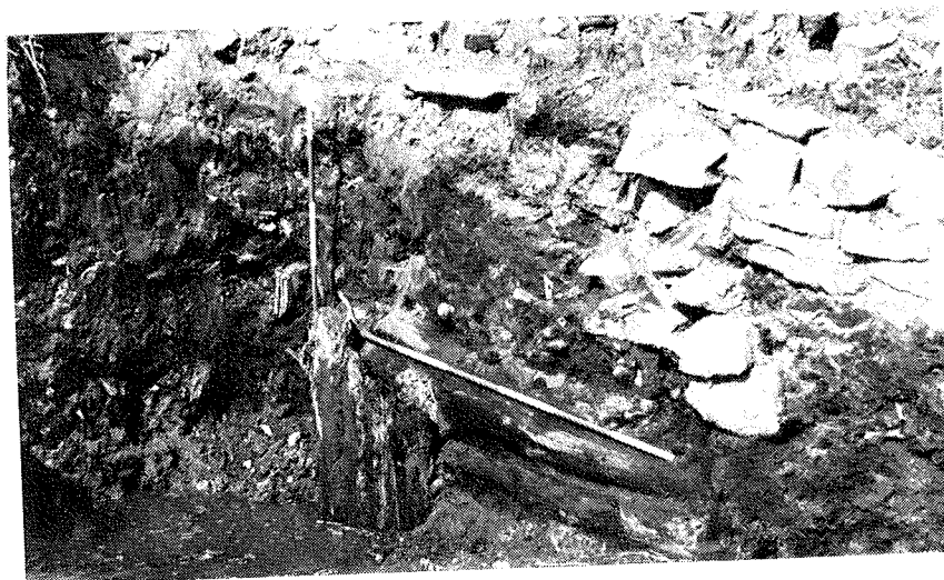
Fig. 47, Kvarteret Vindragaren, mur B. Mur med underliggande rustbädd. Foto mot nordväst. Foto: EJ -79
