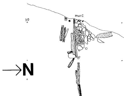
Fig. 64, Kvarteret Vindragaren, anl 4, stensättning, trälämningar. Planritning 1:100 KO -79
