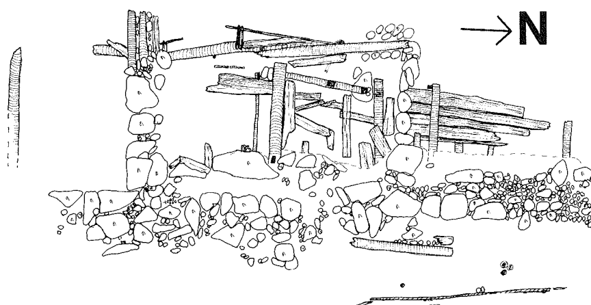
Fig.19, Kvarteret Enigheten, anl 3F. Planritning 1:100 EJ och KO -79
