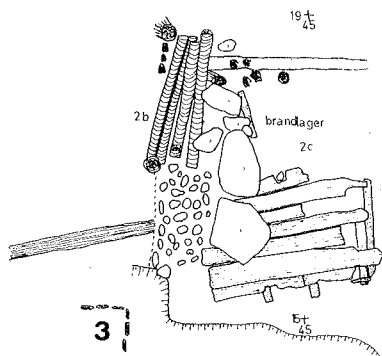
Fig. 61, Kvarteret Vindragaren, anl 2b rustbädd, anl 2c golv (bränt). Planritning 1:100 SK -79.
