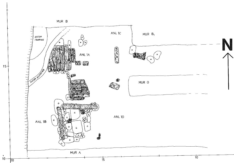
Fig. 11, Kvarteret Enigheten, anl. 1a-1d. Planritning 1:100 EJ -79
