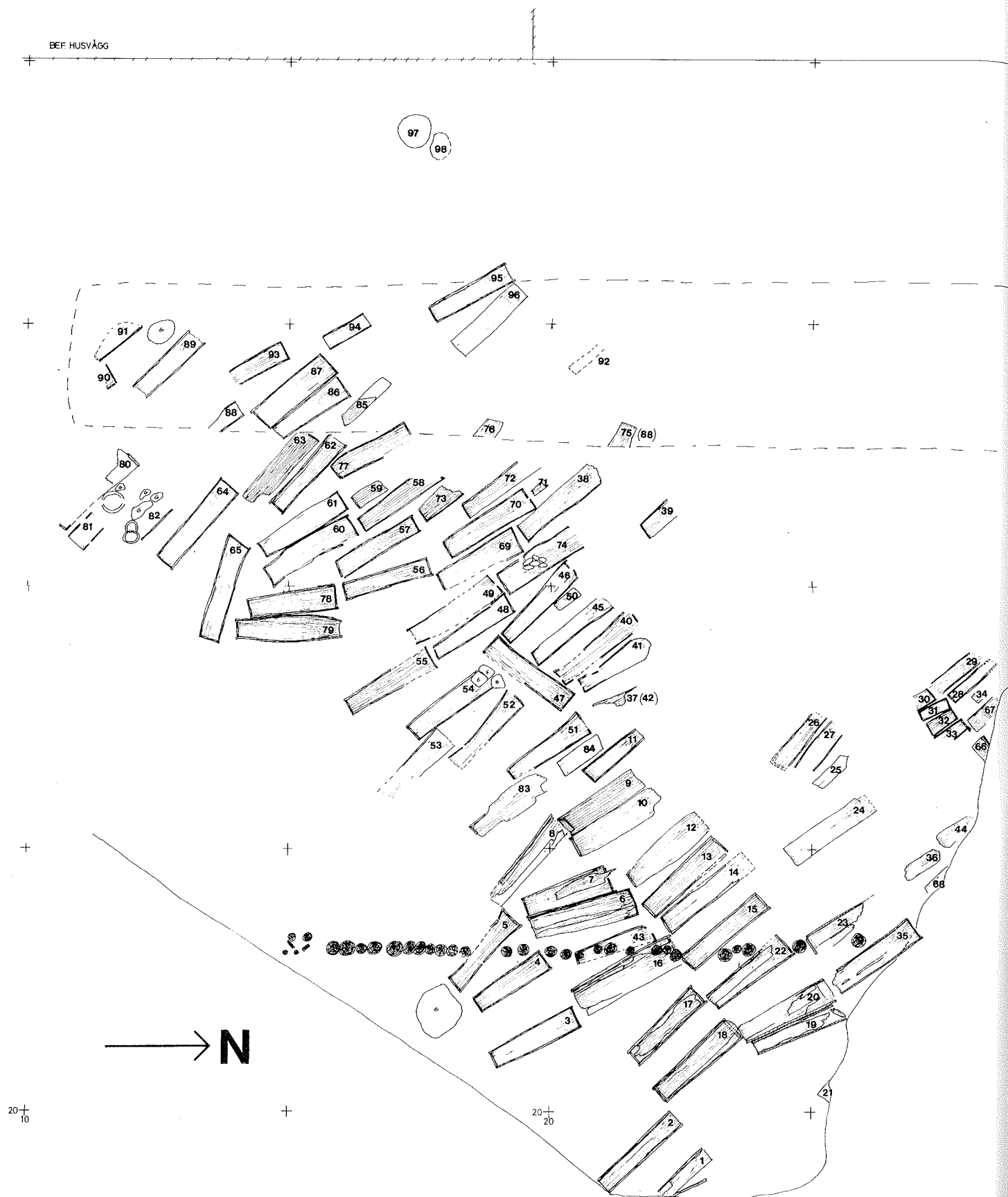
Fig. 82, Kvarteret Vadman, begravningsområdet. Kistor och pålråd. Den streckade linjen markerar profilens läge. Planritning Skala 1:100 EJ, SK, KO -80
