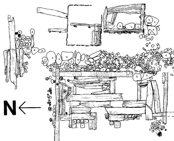
Fig. 17, Kvarteret Enigheten, anl 3B, anl 3E. Avfallsbingar och golv. Planritning 1:100 EJ -79
