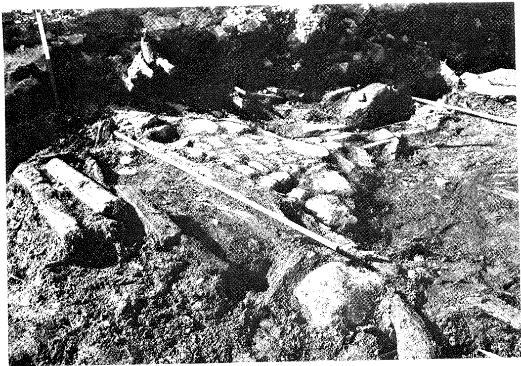
Fig. 65, Kvarteret Vindragaren, anl 4, stenläggning, trälämningar. Foto mot nordväst. Foto: EJ -79
