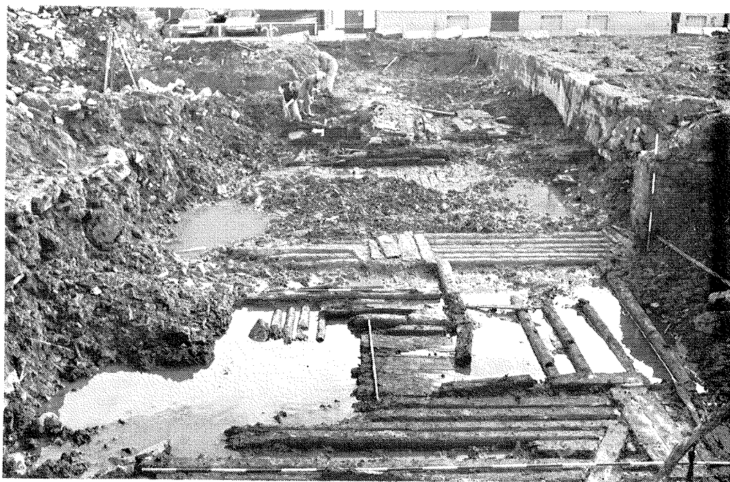
Fig.22, Kvarteret Enigheten, anl 5. Rustbädd. Foto mot söder. Foto: EJ -79
