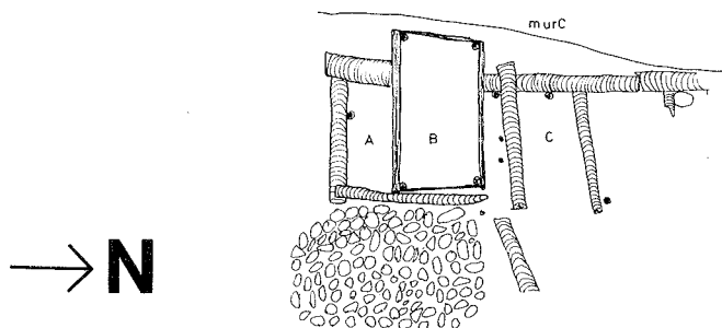
Fig. 67, Kvarteret Vin- dragaren, anl 5 avfallsbingar, stenläggning. Planritning 1:100 KO -79
