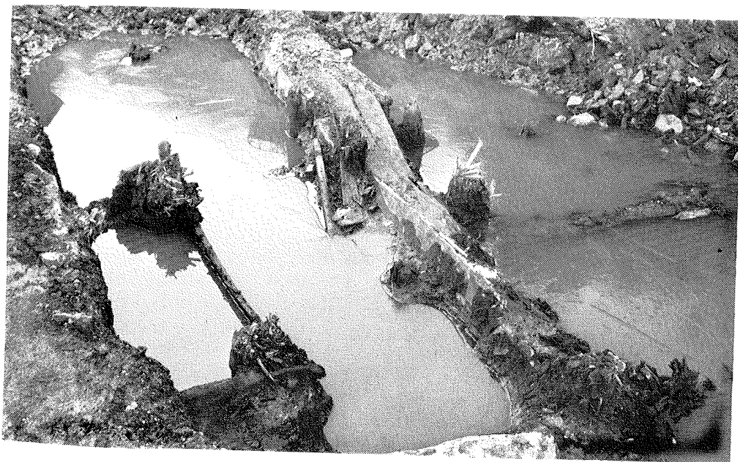
Fig. 26, Kvarteret Enigheten, anl 7. Avfallsbinge och spång. Foto mot nordväst. Foto: EJ -79
