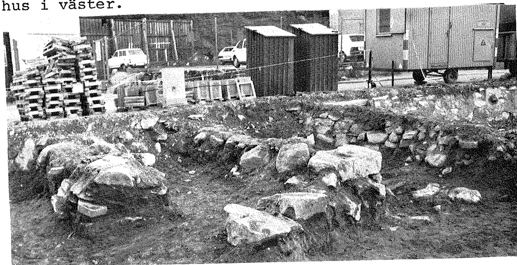
Fig. 33, Kvarteret Enigheten, anl 12-14. Murar. Foto mot nordväst. Foto: EJ -79
