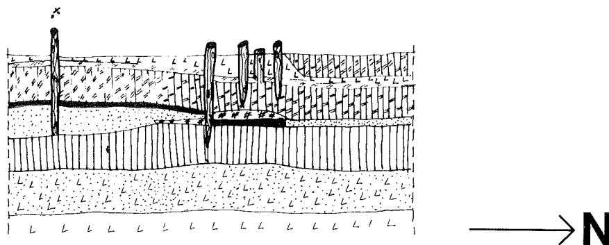
Fig. 10, Kvarteret Enigheten, anl lB, Profilritning mot väster 1:25 EJ-79
