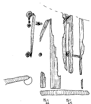
Fig. 62, Kvarteret Vindragaren, anl 2d, träbjälkar under anl 2c. Planritning 1:100 SK -79
