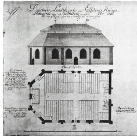
Ritning av "Mariebergskyrkan" utförd år 1786 av Henric Liedin. Det är tveksamt om denna ritning genomfördes. Original i Kungliga Byggnadsstyrelsens arkiv.
