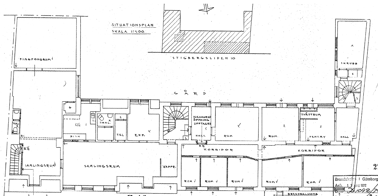
Planritning över övre plan med de förändringar som Kamratföreningen Länkarna gjorde 1972.
