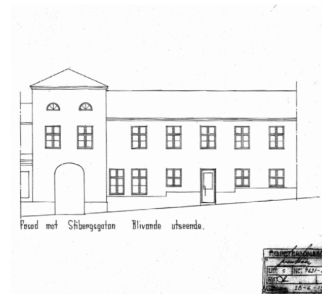
Ritning med upptagen dörr mot Stigbergsgatan år 1943.
