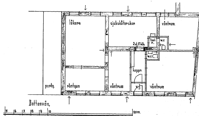
Planritning från 1943 över förändringar som gjordes i läkarmottagningen i den västra byggnadsdelens bottenvåning.
