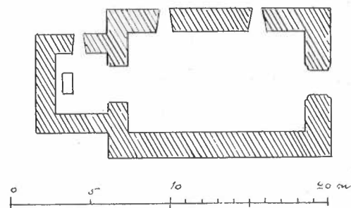
Bild 5. Kyrkans äldsta plan.
