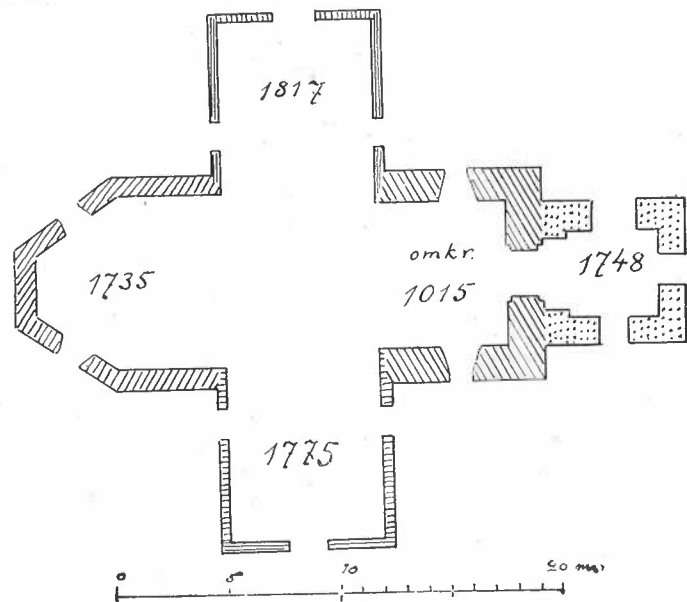
Bild 18. 1817 års (nuvarande) plan.
