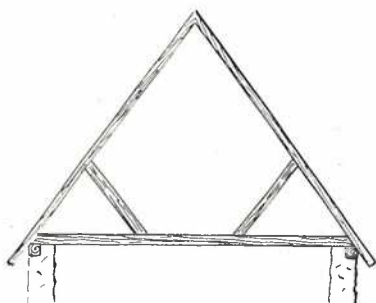
Bild 10. Sparrtakskonstruktion.
