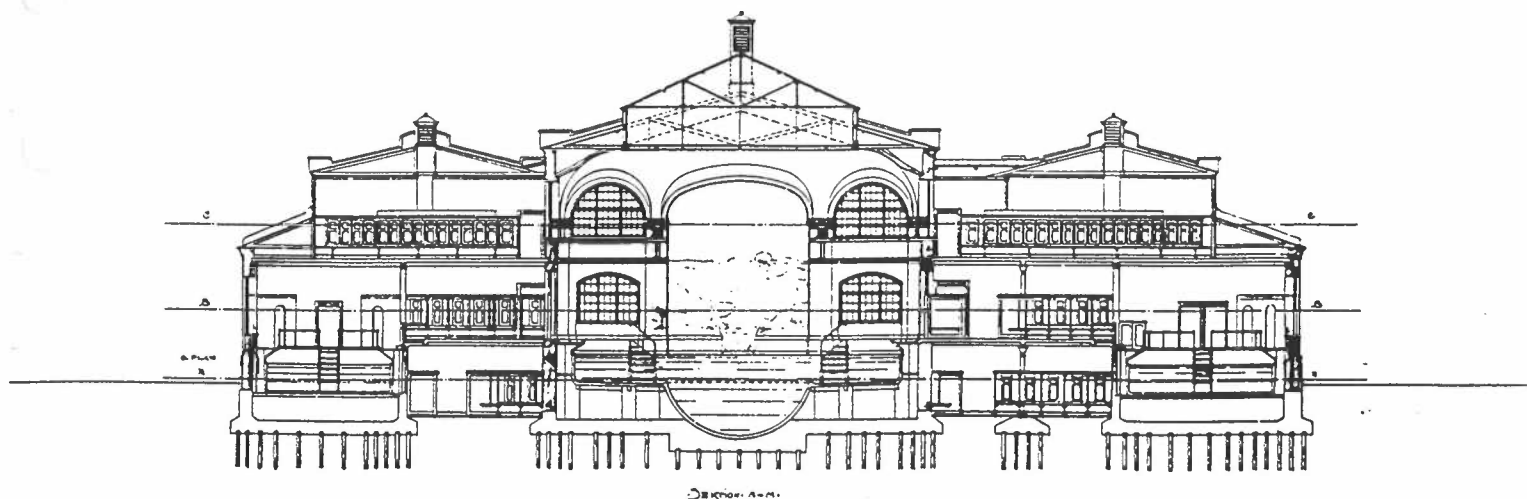
Sektion M-M. Byggnadslovsritning 16 maj 1905. Simhallen sträcker sig genom två-tre våningsplan. Herr- och damavdelningen som omger hallen har omklädningsrum i tre plan och var sin mindre bassäng.
