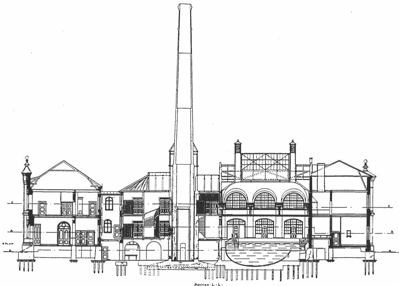
Sektion L-L. Byggnadslovsritning, 16 maj 1905. Simhallens mest karaktäristiska drag är väggarnas stora fönsterpartier, det välv- da taket och bassängens "äggform".
