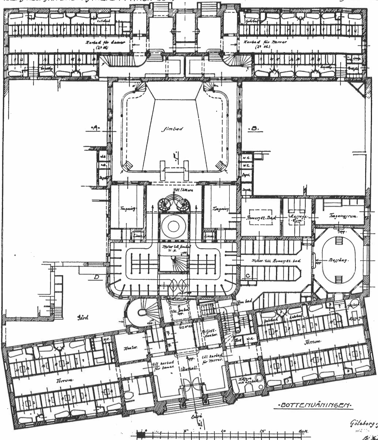
Ombyggnadsritning 1919. Visar nya balkongen och en ny trappa i simhallen samt den delvis ombyggda entré mot Södra Allégatan.
