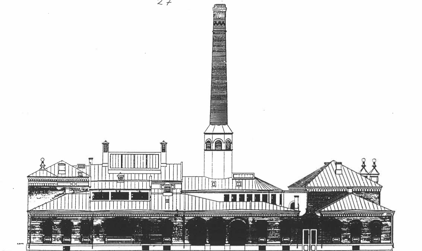
Fasad Kaponjergatan. Byggnadslovsritning, 16 maj 1905.
