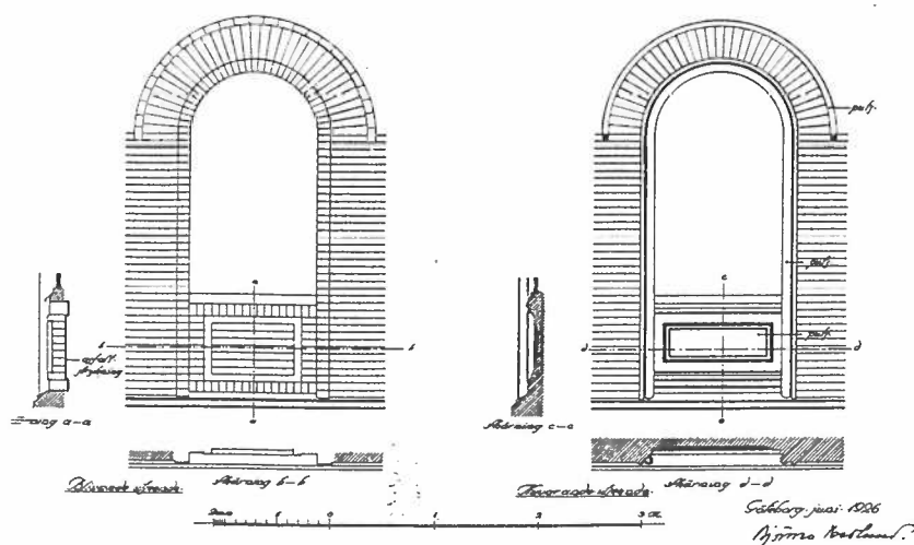
Ombyggnadsritning 1926. Ändring av putspartierna under fönstren till tegelpartier.
