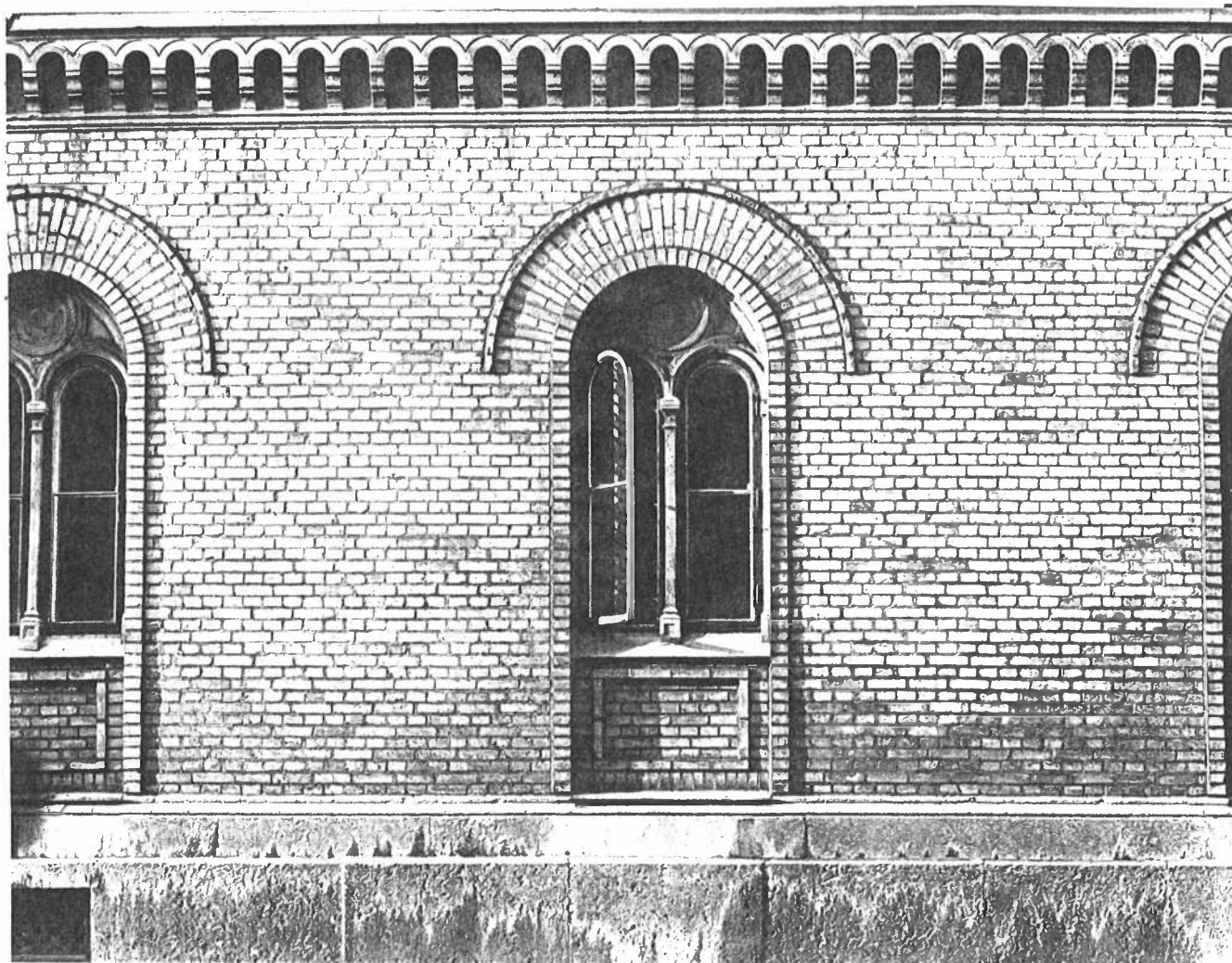
Fasaddetalj som visar den profilerade kalkstenssockeln, fönster med ursprungliga bågar och post i form av kolonn, dekorativ tegelmurning från 1926 och ursprunglig taklist med rundbågemotiv. Foto 1972.
