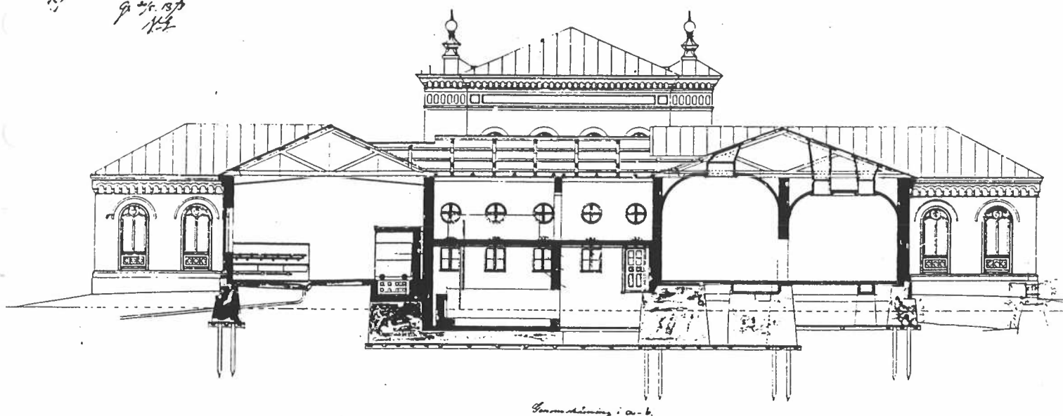
Sektion. Byggnadslovsritning, 30 maj 1873. Observera mellandelens indragning i förhållande till huvudbyggnaden.
