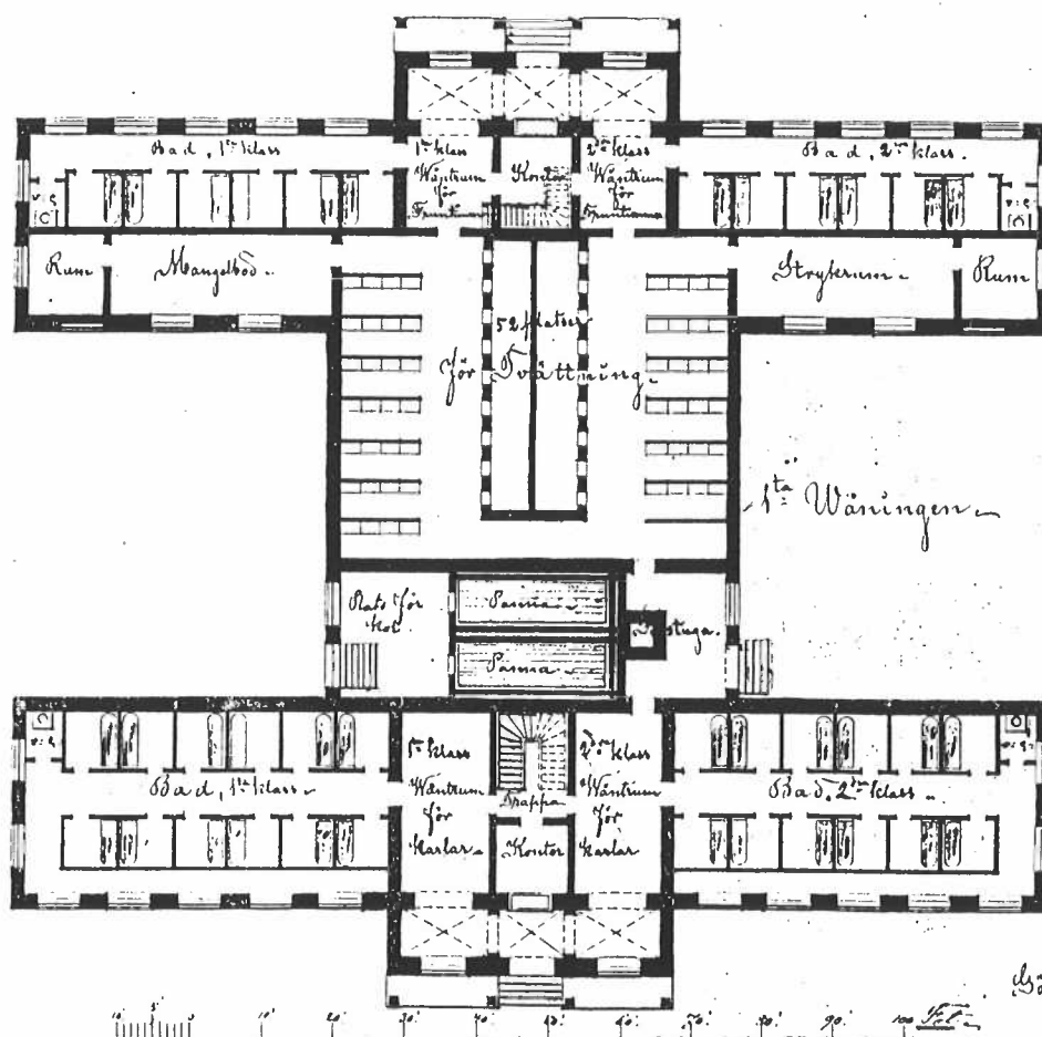
P J Rapps första förslag till badhus, oktober 1870. Observera att badet har en damsida och en herrsida som huvudindelning. Endast karbad finns.
