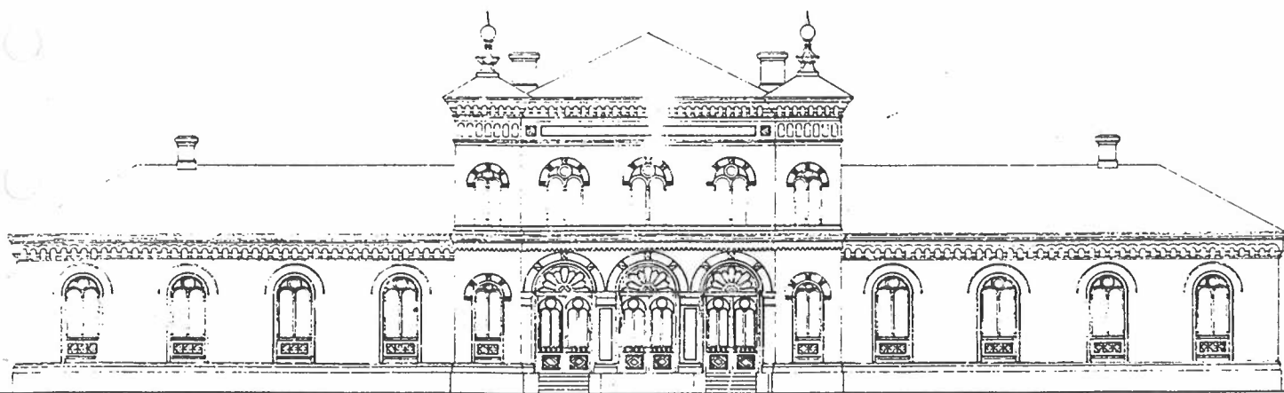
Fasaden mot Haga Östergata. Byggnadslovsritning, 30 maj 1873. Fasaden har samma utseende idag med undantag av entrédörrarna.
