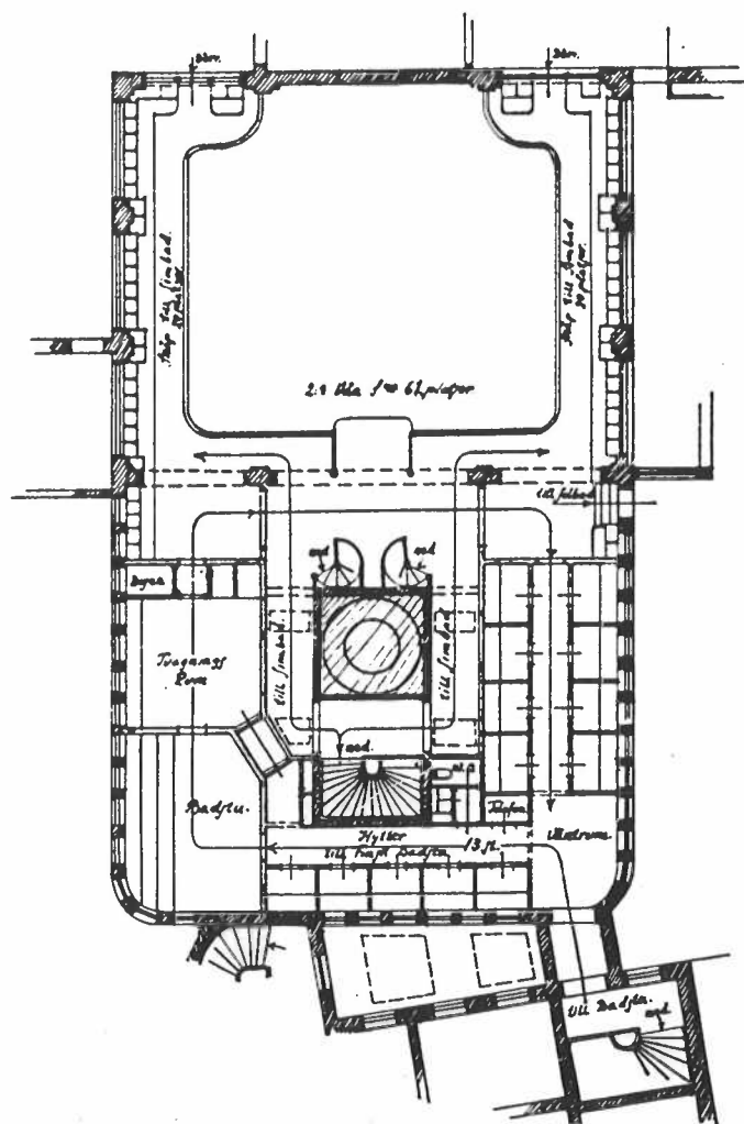
Ombyggnadsritning 1919. Visar simhallens övre plan med klädska på den nya balkongen samt ombyggnad för bastu i en del av fd omklädningsrummen.
