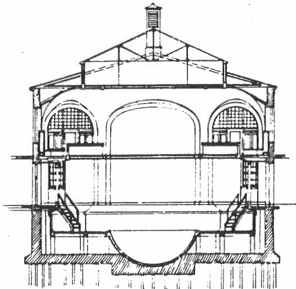
SKÄRNING A-D.
