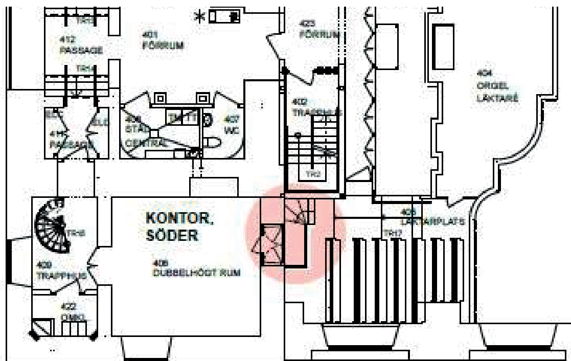
Dörr och trappa vid orgelläktaren efter ombyggnad. Ritning DFYRA arkitekter ab. Pardörren har flyttats och livar väggen på orgelläktaren, inåt kontorsrummet sitter en ny dörr och trappan ner till orgelläktaren har flyttats ut på läktaren.
