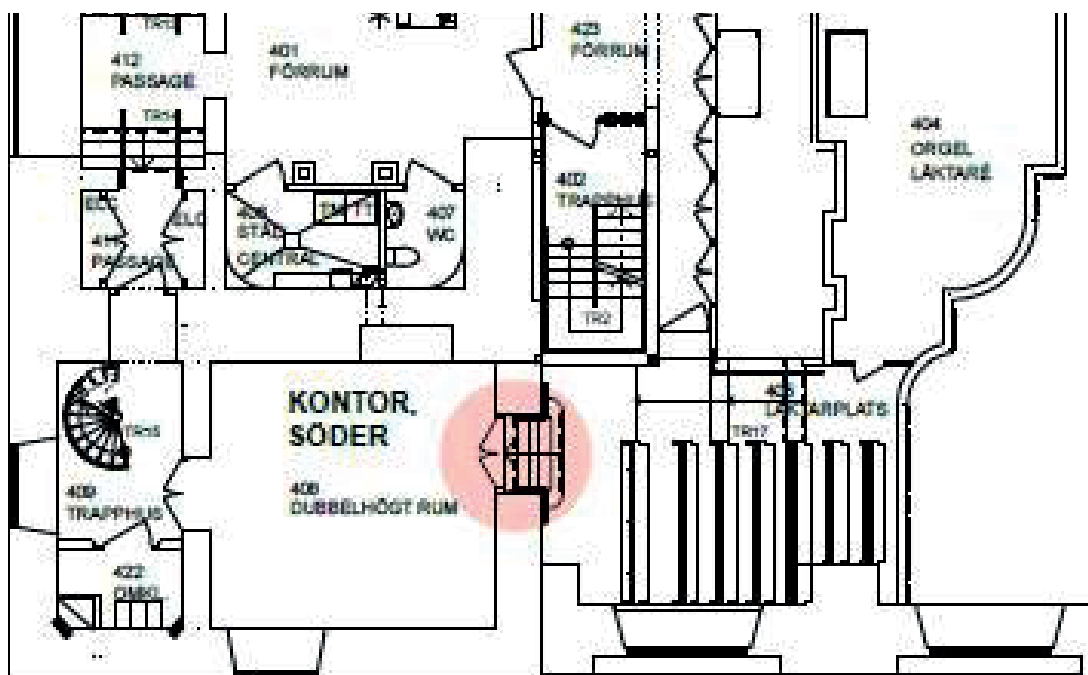
Dörr och trappa vid orgelläktaren före ombyggnad. Ritning DFYRA arkitekter ab. Pardörren livar kontorsrummets vägg och trappans fem steg ner till läktaren börjar i muröppningen. Stegen är av ek.
