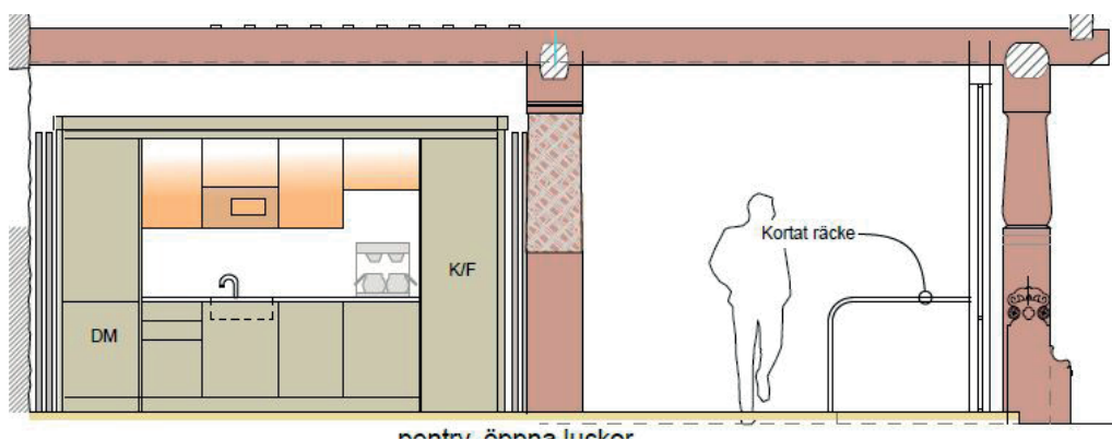
Skissen visar pentryt och den ledstång som stödjer steget mot den bakre dörren. Fotot visar den kortade ledstången och det kompletterade golvet.
