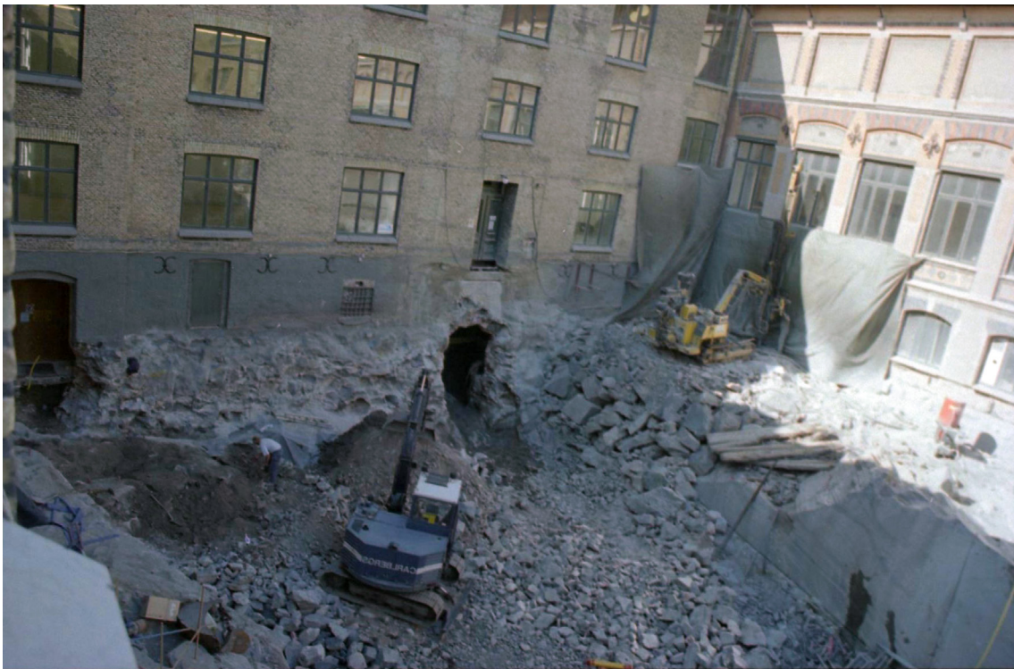
Figur 19. Innergården vid urschaktning av sprängt berg efter att lämningarna avlägsnats, mot nordväst.
