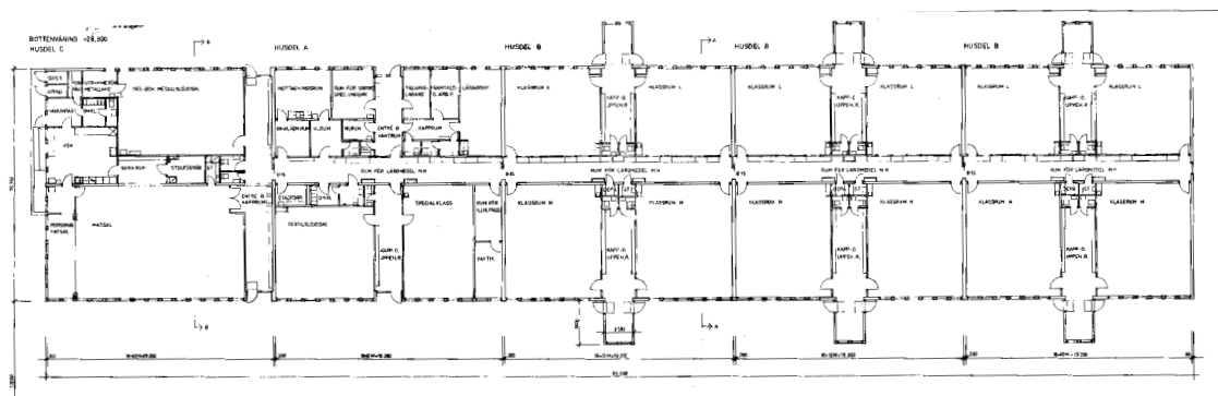
Planritning över Brudbergsskolans klassrumsbyggnad, daterad år 1968. Skolan byggdes efter Skolöverstyrelsens BASK-typitritningar.
