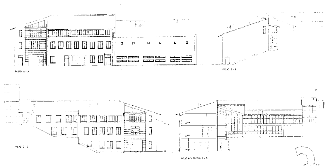
Fasadritningar för Katolska skolan, daterade år 1995. GF arkitekter ritade den stora nybyggnaden, som slingrar sig i en typ av S-form uppför sluttningen på västra sidan av Danska Vägen.
