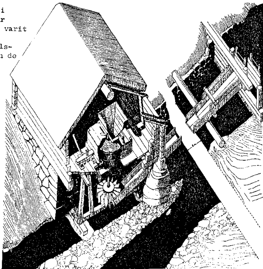
Skvaltkvarnens konstruktion. Efter Kulturen 1938
