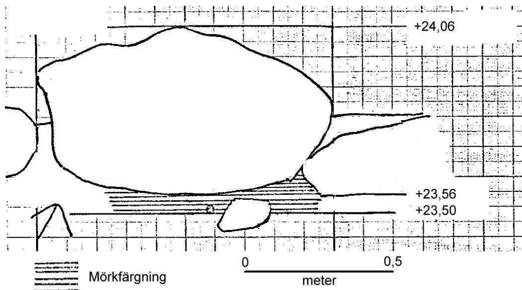
Anläggning 4 Profil B-A
