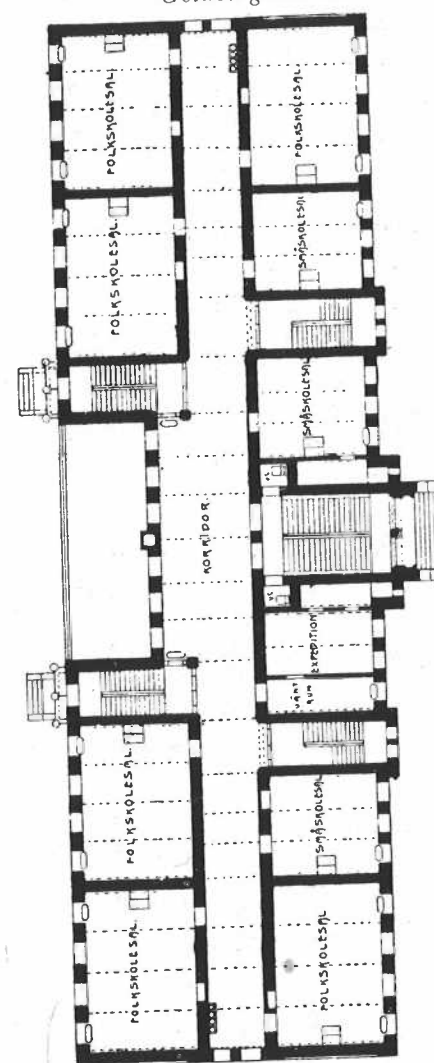
Plan av bottenvåningen
