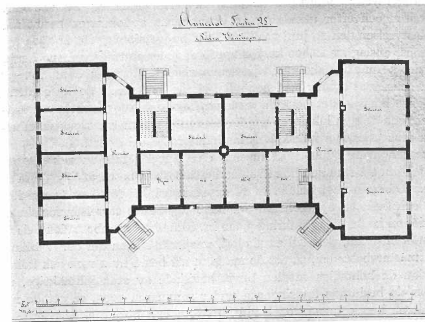
Plan av nedre våningen
