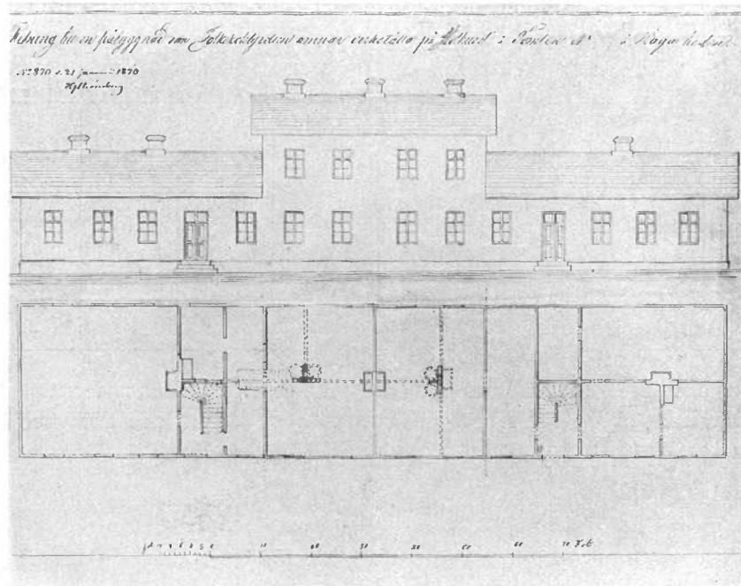
Hagahedens skolhus, efter ritning
