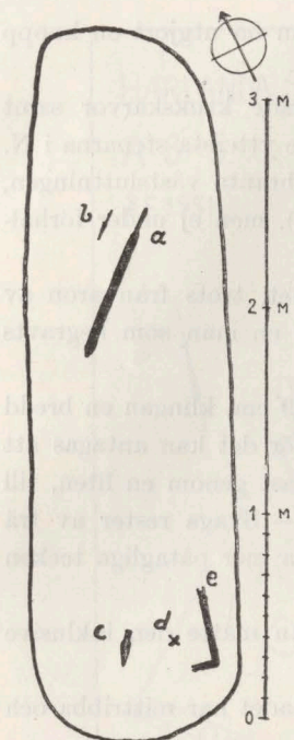
Fig. 3. Gravgropen i A 2 med svärd (a), kniv (b), spjutspets (c), hartstättning (d) och spår av träkista (e).
