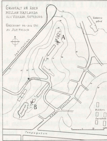
Fig. 7. Karta över gravfält A och B i Härlanda. Av bebyggelsen på åsen har endast de närmast gravfälten belägna huslängorna angetts.
