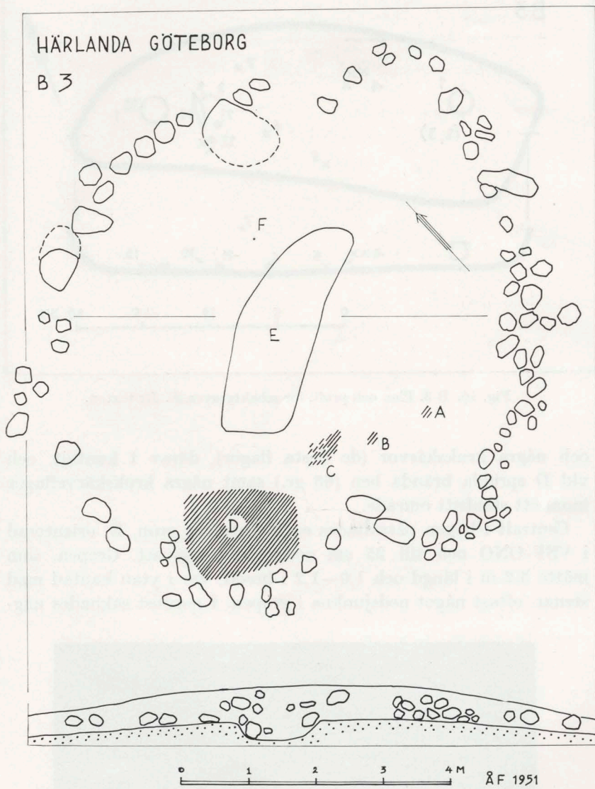
Fig. 15. B 3. Plan och profil. För beteckningar se text.
